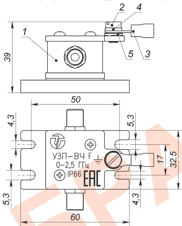
Рис.1 Состав и габаритно-установочные размеры (позиции смотри комплект поставки)
